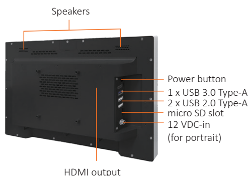
HDMI output
